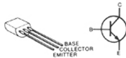
2SC383TM Q9
