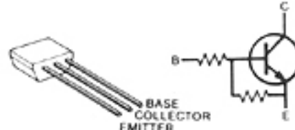
RN1202 Q1
