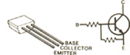
RN1202 Q104
