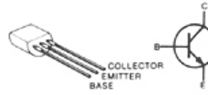
2SC2026 Q18
