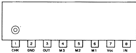
HD10551 (PRESCALER)
